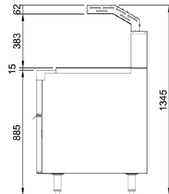
End Elevation
